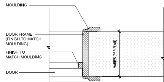
(B) SIDE JAMB SECTION
