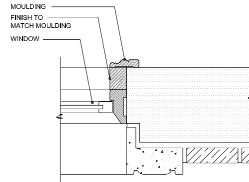
(B) SIDE JAMB SECTION
